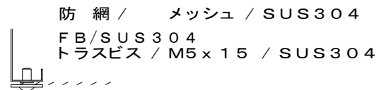
網 詳細図
