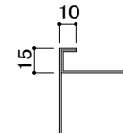
天板部詳細
