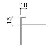
天板部詳細
